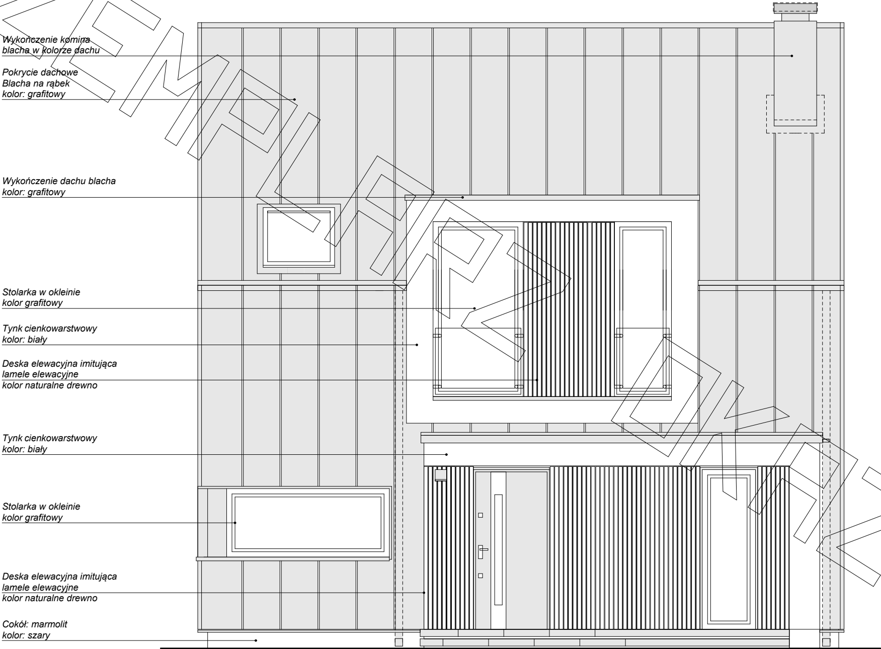
ELEWACJA FRONTOWA
