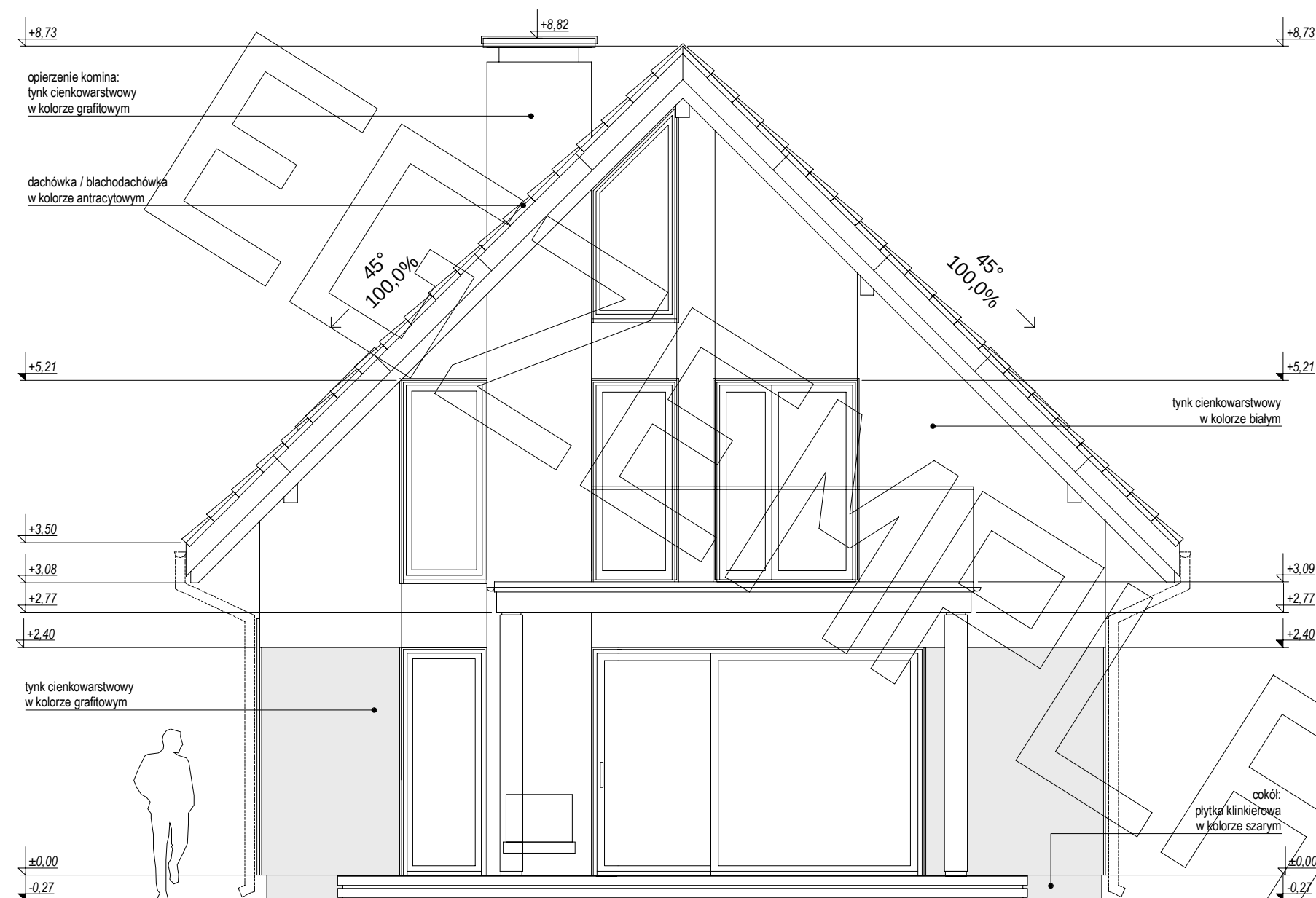
ELEWACJA TYLNA
